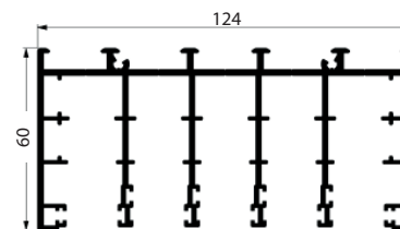
Profilo superiore 5 ante Upper frame 5 rails
