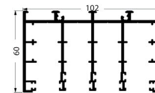
Profilo superiore 4 ante Upper frame 4 rails
