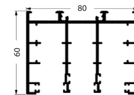
Profilo superiore 3 ante Upper frame 3 rails
