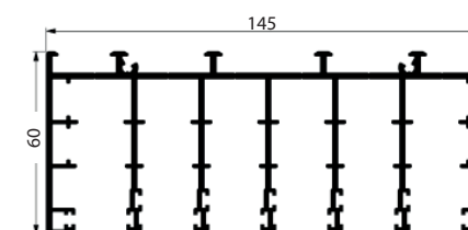
Profilo superiore 6 ante Upper frame 6 rails
